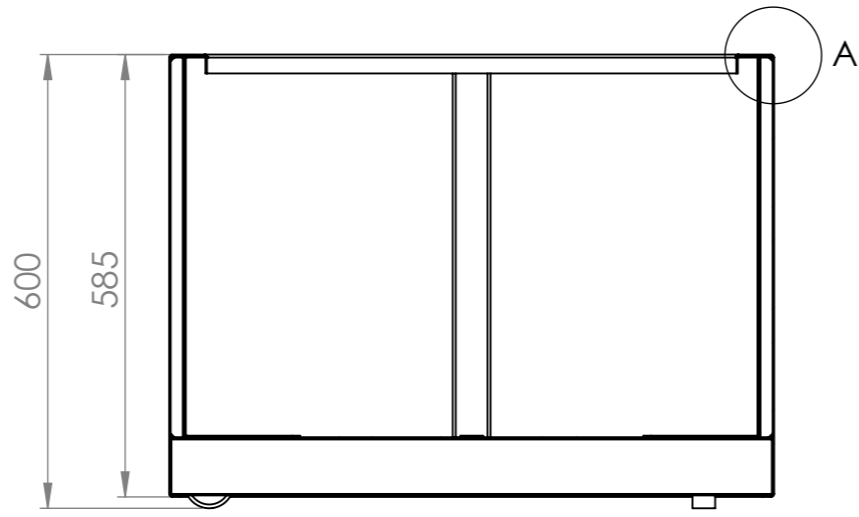
SECTION B-B SKALA 1 : 10
